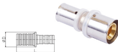
Reducing Union · 异径直通
