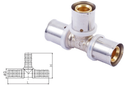
Equal Tee · 等径三通
