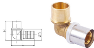
Copper Elbow · 接紫铜管弯头
